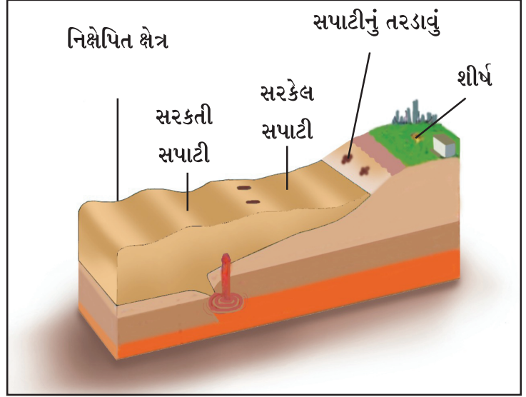
ભૂસ્ખલન-પ્રક્રિયા
